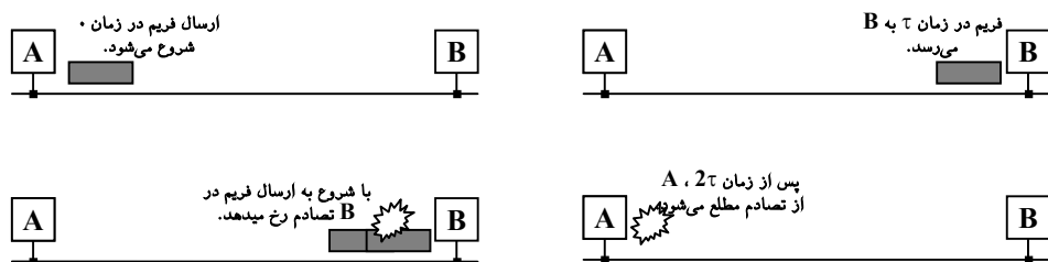
شکل (۶-۲) مراحل کشف تصادم
