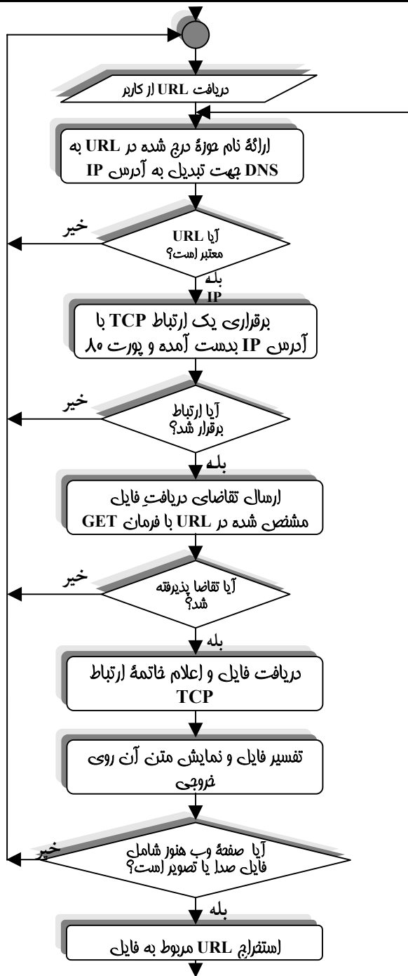
شکل (۳-۱۰) فلوچارت عملیات مرورگر برای دریافت یک صفحه وب
