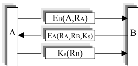
شکل (۱۱-۱۱) احراز هویت با استفاده از کلید عمومی و روش RSA
