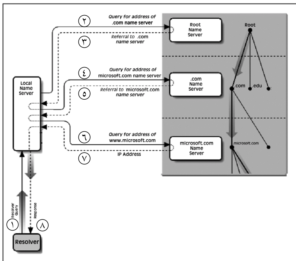
شکل (۱-۶) روند ترجمه نام به روش پرس و جوی تکراری
