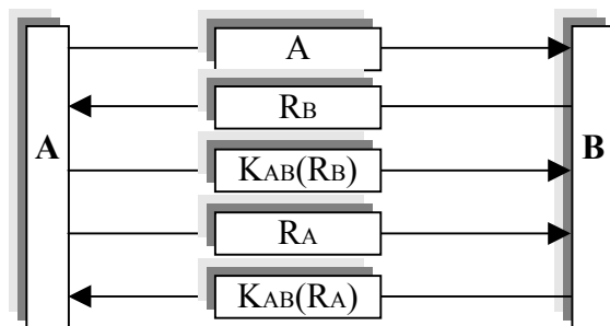
شکل (۱۰-۱۱) احراز هویت با کلید مشترک
